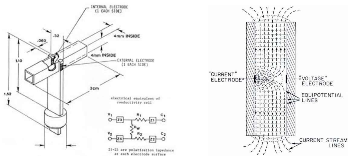
Рисунок 1. – Схема кондуктивной 4х-электродной ячейки NBIS и распределение силовых линий в ней.
