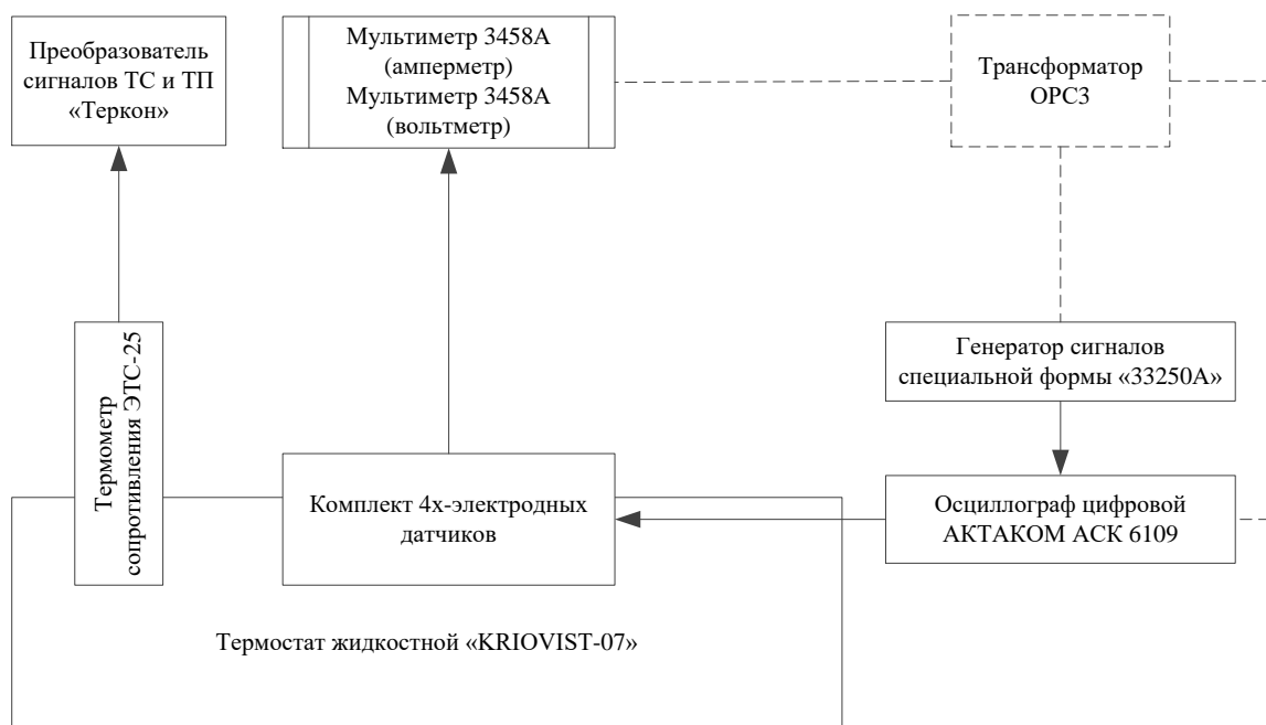
Рисунок 3 – Схема установки
