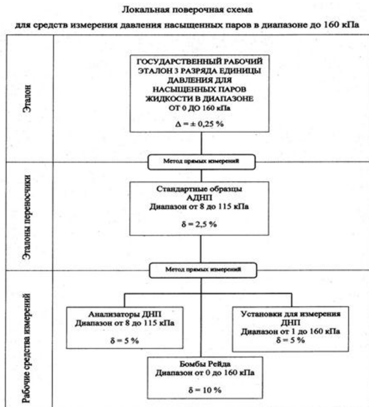
Рисунок 4 - проект локальной поверочной схемы для СИ ДНП
