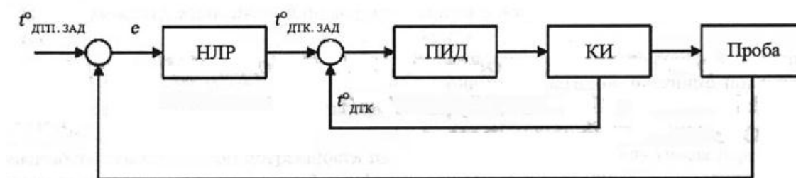
Рисунок 6 - Структура ПИД регулятора
